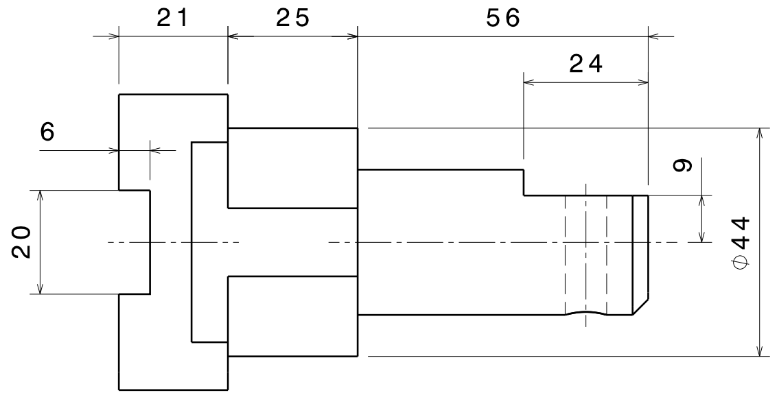
Vue de face Echelle : 1:1
