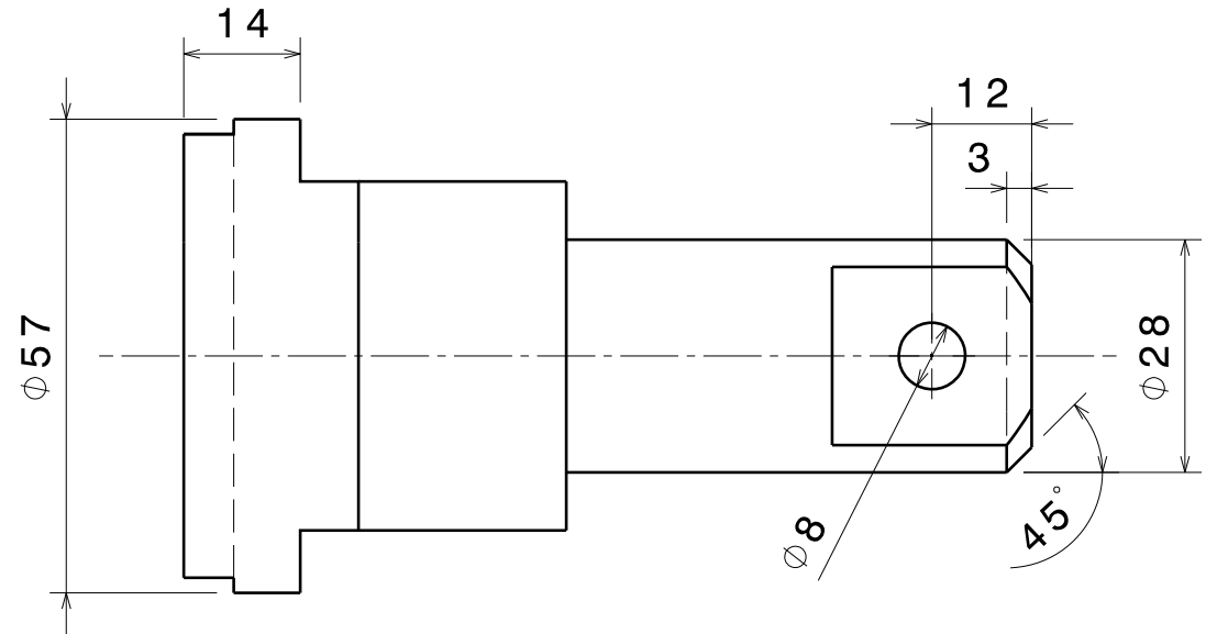
Vue de face Echelle : 1:1
