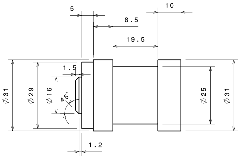
Vue de face robinet Echelle : 1:1
